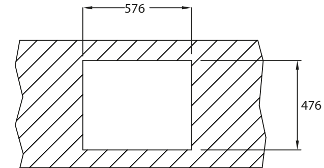
Hueco para encastre Fitting hole for inset sink
